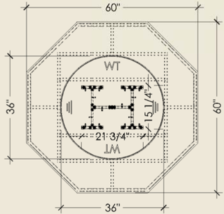
TOP ELEVATION
